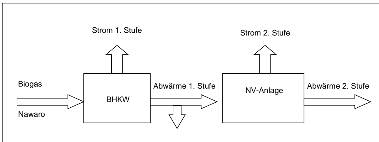
Abbildung 1: Zweistufige Verstromung mit Nachverstromung (NV)
