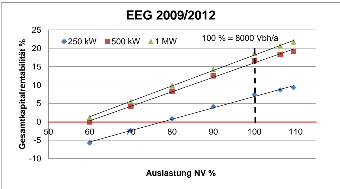
Abbildung 5: Einfluss der Auslastung der NV in % auf die Gesamtkapitalrentabilität getrennt nach BHKW Leistung (250, 500, 1.000 kW) als Mittelwert der EEG 2009 und 2012 bei einem Jahresnutzungsgrad der NV von 8 % und einer Nutzungsdauer von 10 Jahren.
