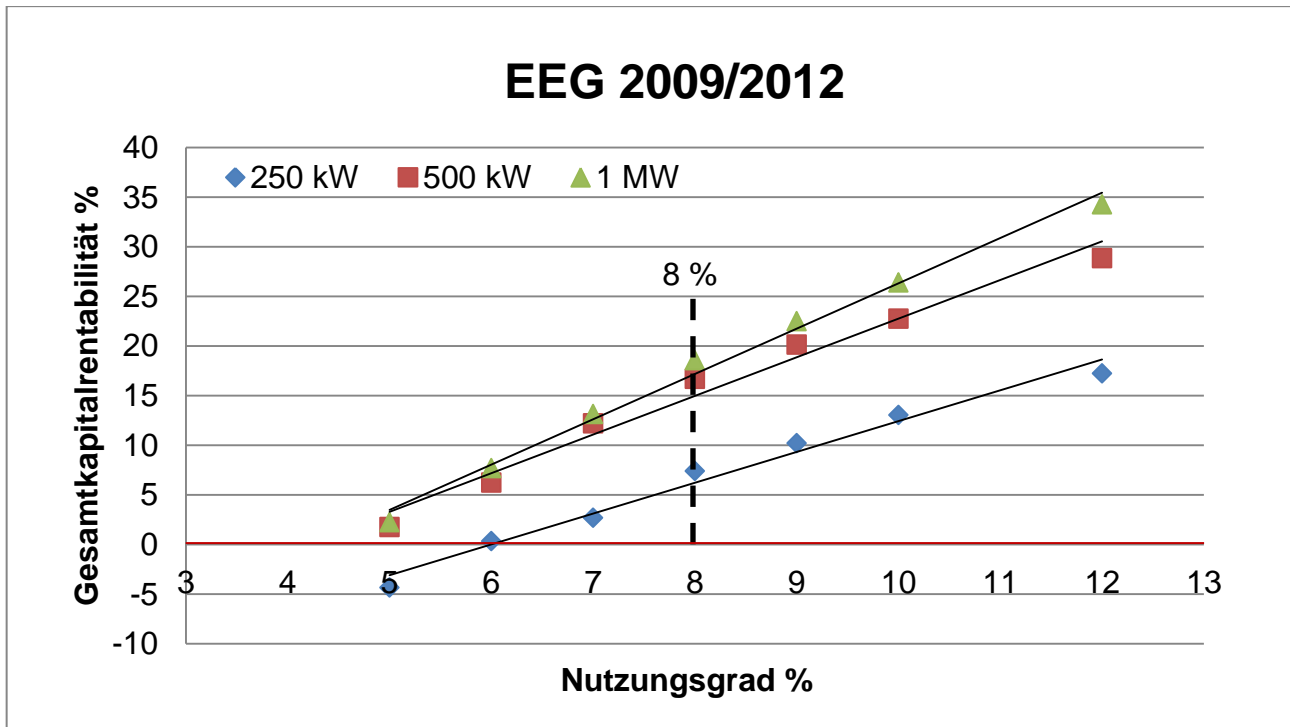
Abbildung 3: Einfluss der Variation des Jahresnutzungsgrads auf die Gesamtkapitalrentabilität getrennt nach BHKW Leistung (250, 500, 1.000 kW) als Mittelwert der EEG 2009 und 2012 bei einer Nutzungsdauer der NV von 10 Jahren.
