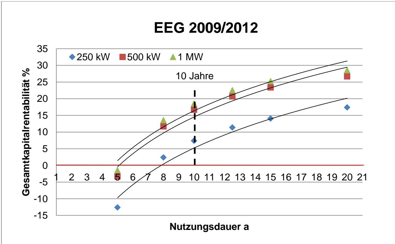
Abbildung 4: Einfluss der Variation der Nutzungsdauer auf die Gesamtkapitalrentabilität getrennt nach BHKW Leistung (250, 500, 1.000 kW) als Mittelwert der EEG 2009 und 2012 bei einem Jahresnutzungsgrad der NV von 8 %.
