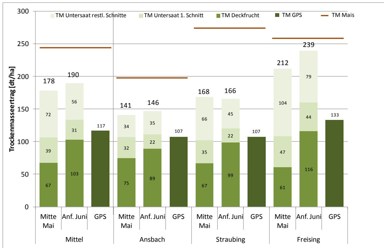
Abb.1: Trockenmasseertrag von Deckfrucht (DF) Winterroggen und Untersaat Weidelgras (WD) zu 2 GPS-Erntezeitpunkten (Mitte Mai bzw. Anf. Juni) im Vergleich zum alleinigen GPS-Anbau und Hauptfruchtmais in Abhängigkeit vom Standort (Mittel 2007-2010)
