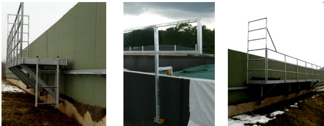
Abb. 14 - 16: Außen oder an der Krone: verschiebbare Varianten sind möglich, müssen jedoch immer an der möglichen Absturzstelle vorhanden sein.
